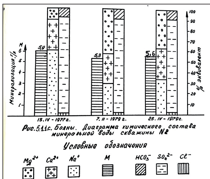
Рис. № 3. Діаграма хімічного складу мінеральної води свердловини № 2.
